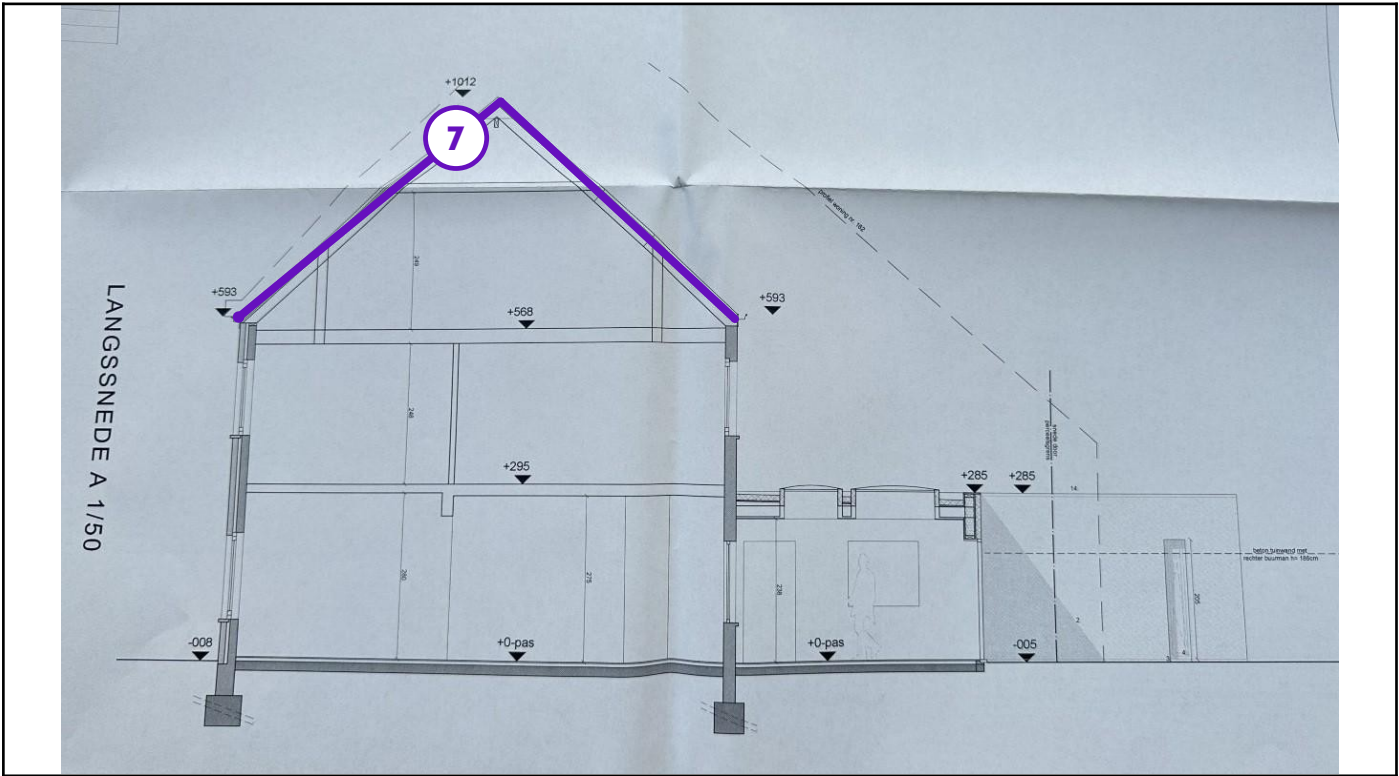
Legende van plan 1.9: doorsnede onderdak
